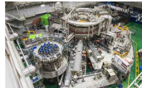
Reactor KSTAR Fuente: Consejo Nacional de Investigación de Ciencia y Tecnología de Corea del Sur
