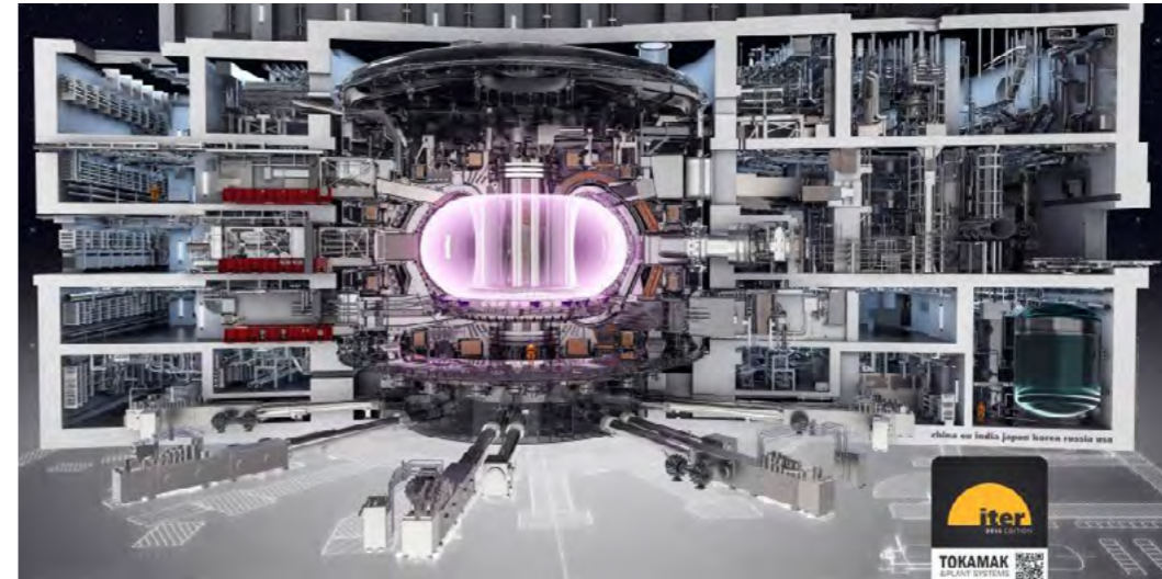
Reactor con forma de Tokamak Fuente: ITER
